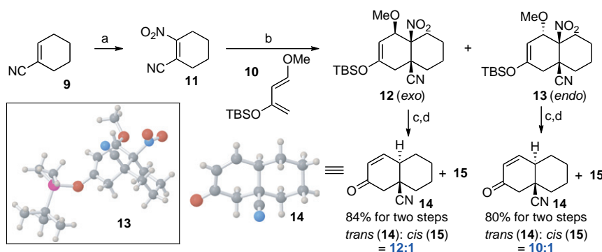
Scheme 1. Reagents and conditions: (a) \text{NaNO}_2 , CAN, \text{CH}_3\text{CN} , rt, 24 h, 56%; (b) toluene, 100^\circ\text{C} , 80 h, 78%; (c) n\text{-Bu}_3\text{SnH} , AIBN, benzene, reflux, 2 h; (d) HF, \text{CH}_3\text{CN} , 1 h.
